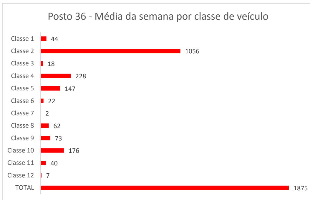
Gráfico 240: Média da semana por classe de veículo no Posto 36.
