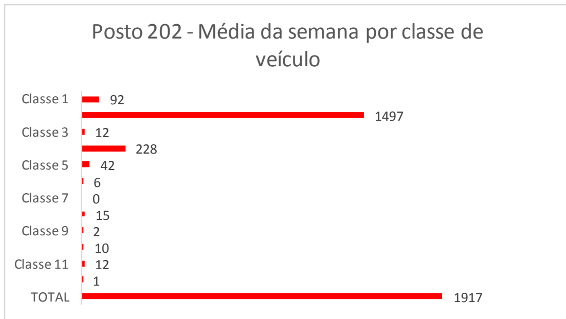
Gráfico 478: Média da semana por classe de veículo no Posto 202.
