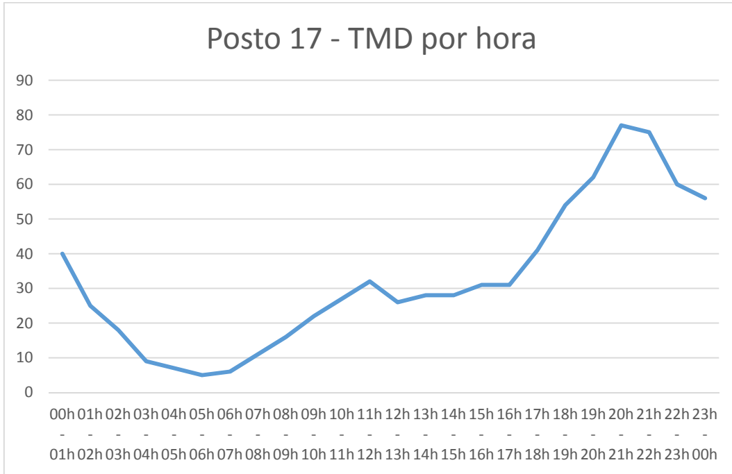
Gráfico 552: Tráfego médio diário (TMD) por hora no Posto 17.
