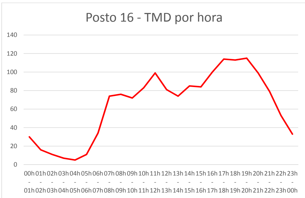
Gráfico 517: Tráfego médio diário (TMD) por hora no Posto 16.
