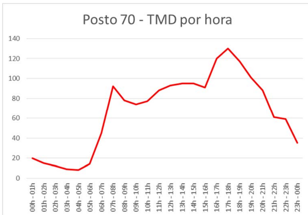
Gráfico 105: Tráfego médio diário (TMD) por hora no Posto 70.
