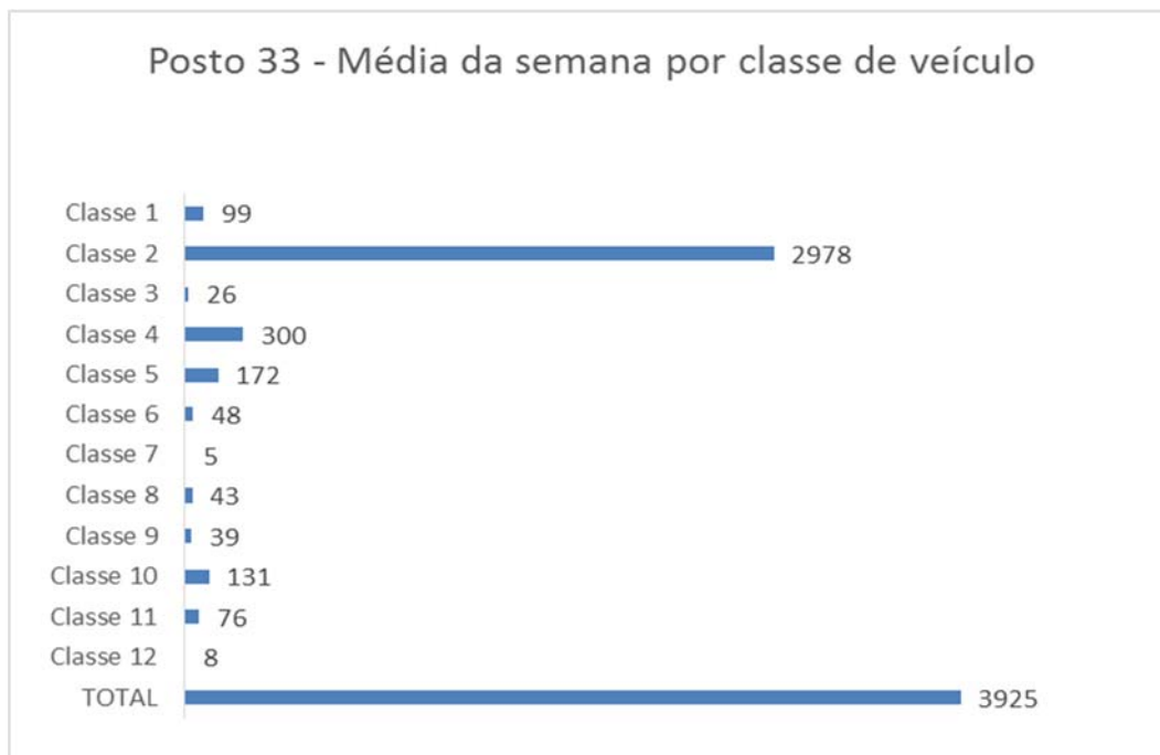
Gráfico 204: Média da semana por classe de veículo no Posto 33.
