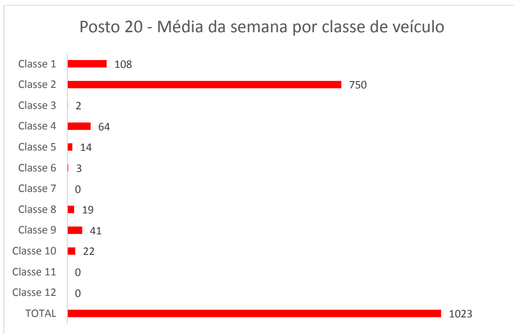
Gráfico 577: Média da semana por classe de veículo no Posto 20.
