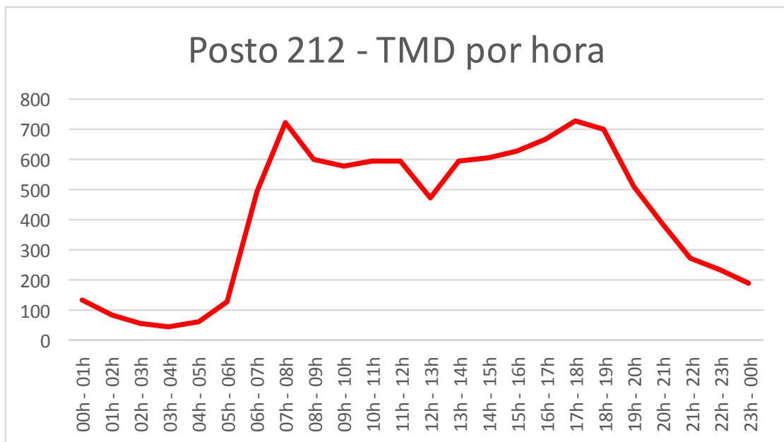
Gráfico 634: Tráfego médio diário (TMD) por hora no Posto 212.
