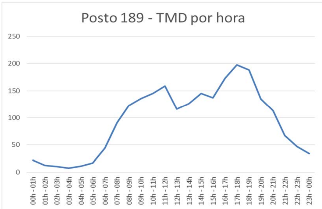
Gráfico 167: Tráfego médio diário (TMD) por hora no Posto 189
