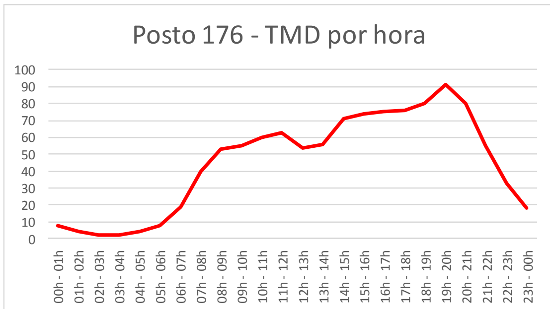
Gráfico 622: Tráfego médio diário (TMD) por hora no Posto 176.
