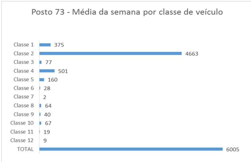
Gráfico 429: Média da semana por classe de veículo no Posto 73.
