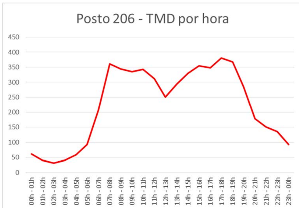
Gráfico 274: Tráfego médio diário (TMD) por hora no Posto 206.
