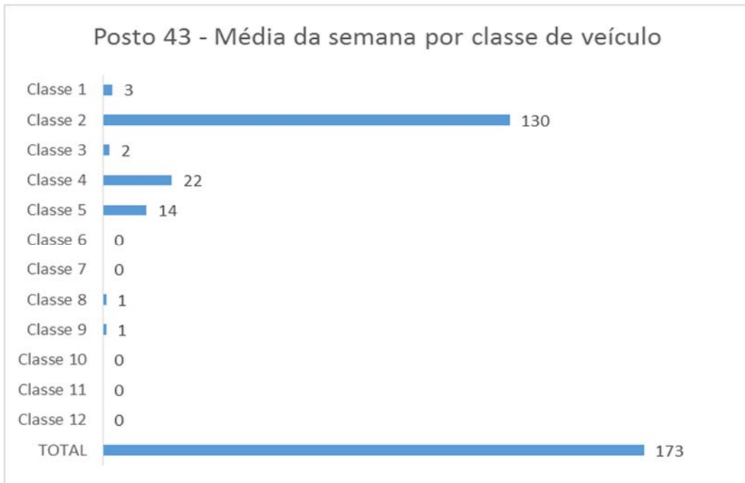
Gráfico 074: Média da semana por classe de veículo no Posto 43.
