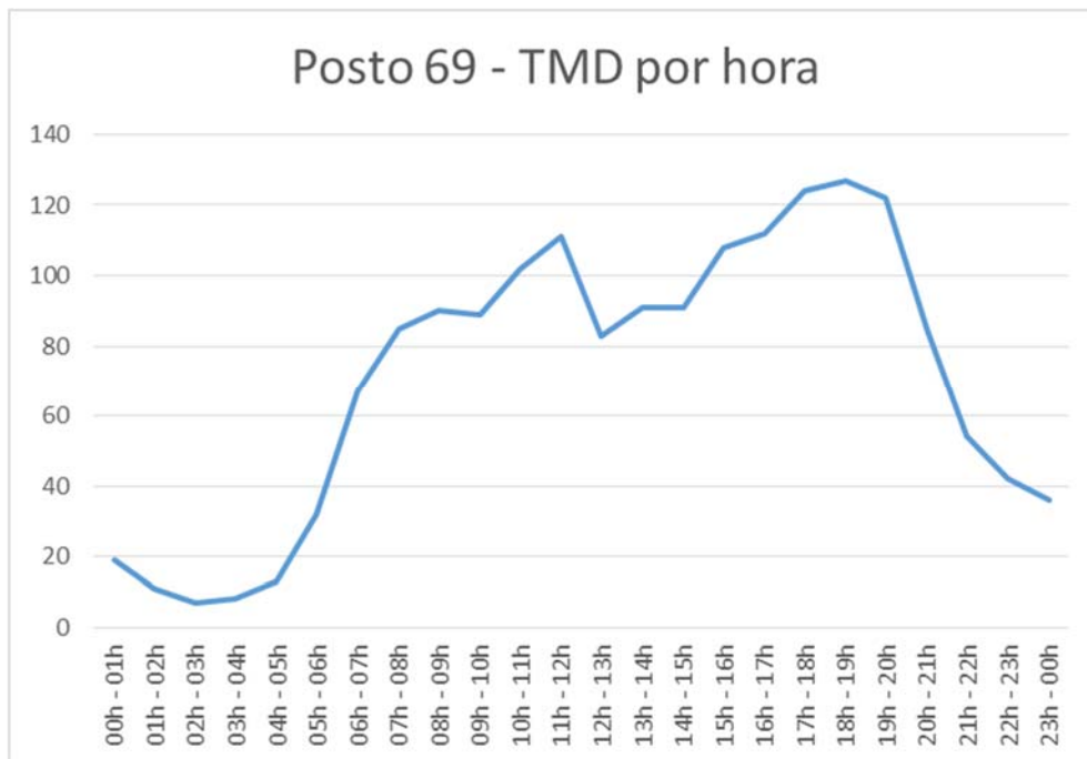
Gráfico 104: Tráfego médio diário (TMD) por hora no Posto 69.
