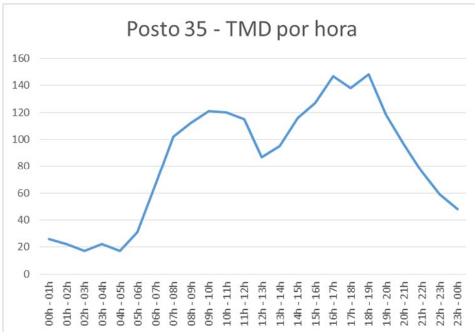
Gráfico 237: Tráfego médio diário (TMD) por hora no Posto 35.
