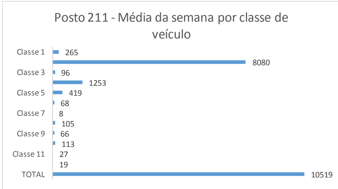
Gráfico 635: Média da semana por classe de veículo no Posto 211.
