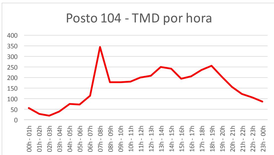
Gráfico 606: Tráfego médio diário (TMD) por hora no Posto 104.
