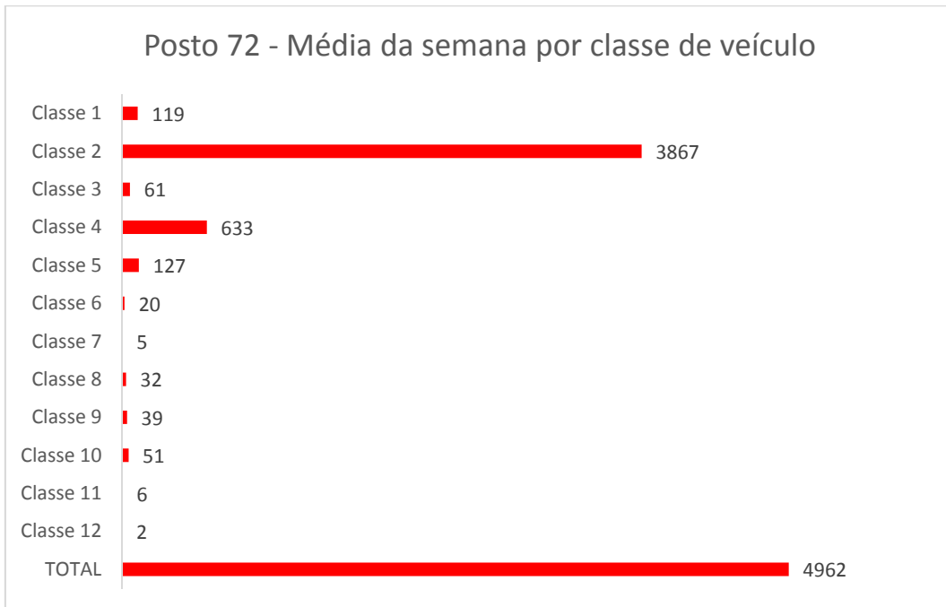
Gráfico 150: Média da semana por classe de veículo no Posto 372
