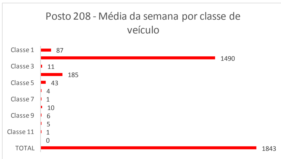
Gráfico 628: Média da semana por classe de veículo no Posto 208.
