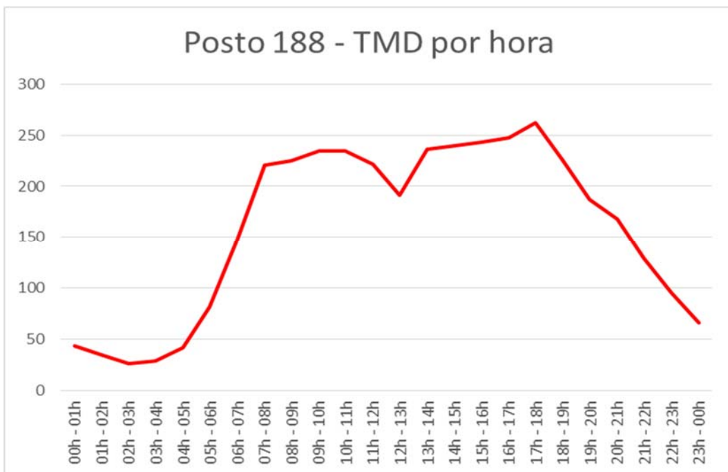
Gráfico 164: Tráfego médio diário (TMD) por hora no Posto 188
