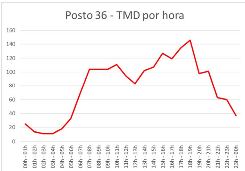
Gráfico 238: Tráfego médio diário (TMD) por hora no Posto 36.
