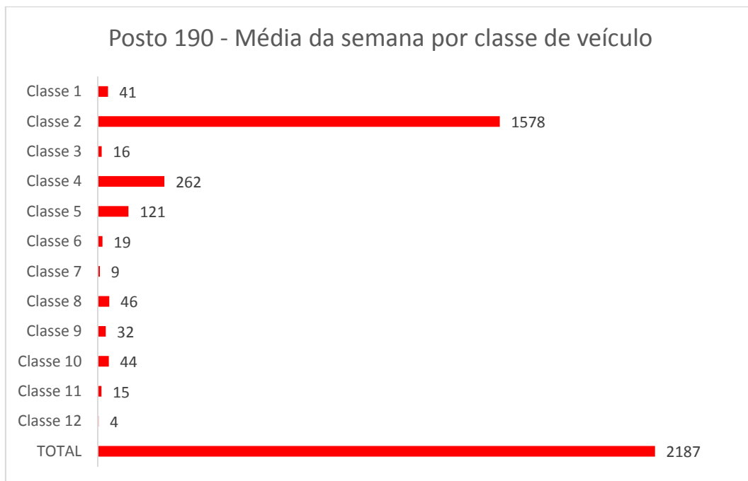
Gráfico 170: Média da semana por classe de veículo no Posto 190
