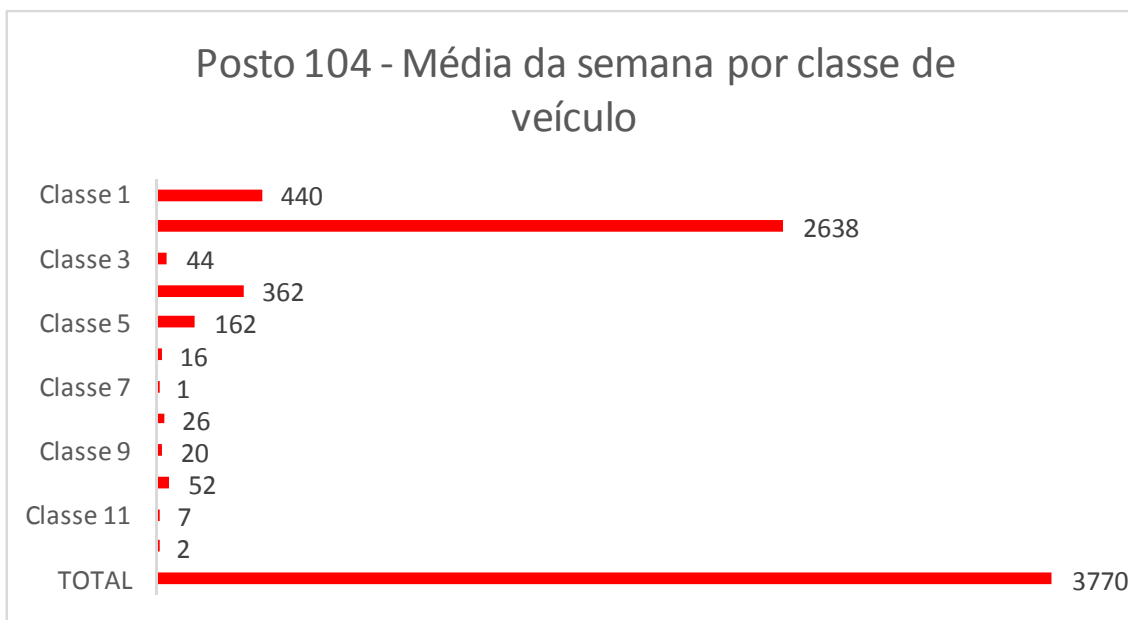
Gráfico 608: Média da semana por classe de veículo no Posto 104.
