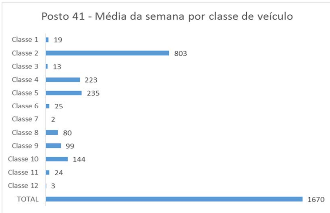
Gráfico 039: Média da semana por classe de veículo no Posto 41.
