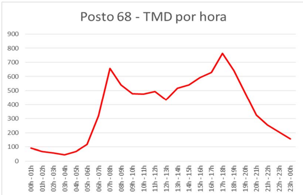
Gráfico 144: Tráfego médio diário (TMD) por hora no Posto 68
