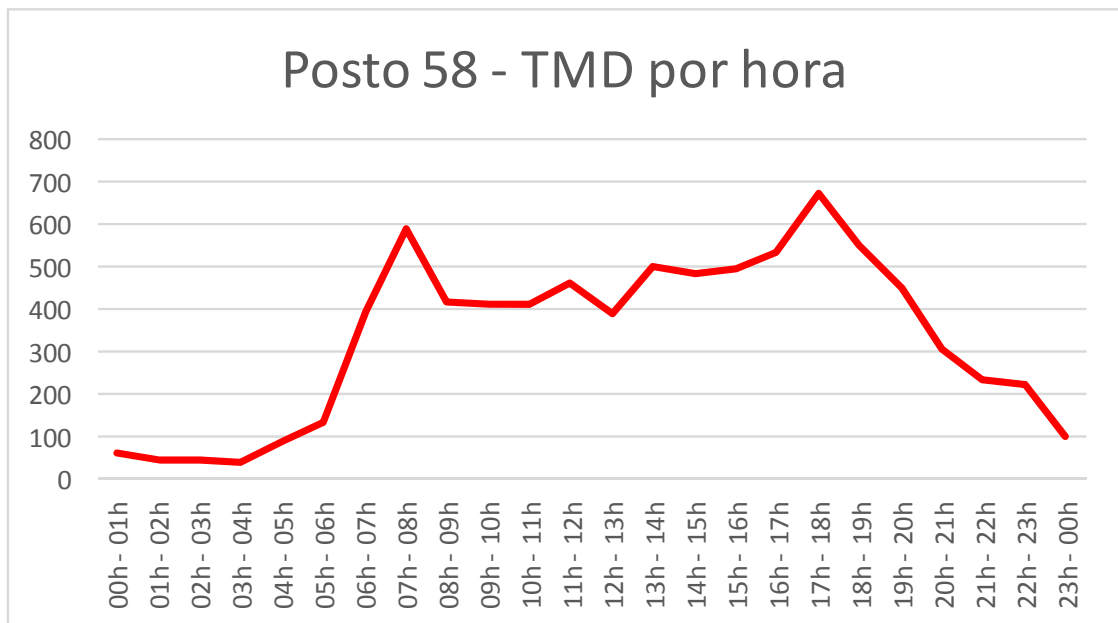
Gráfico 424: Tráfego médio diário (TMD) por hora no Posto 58.
