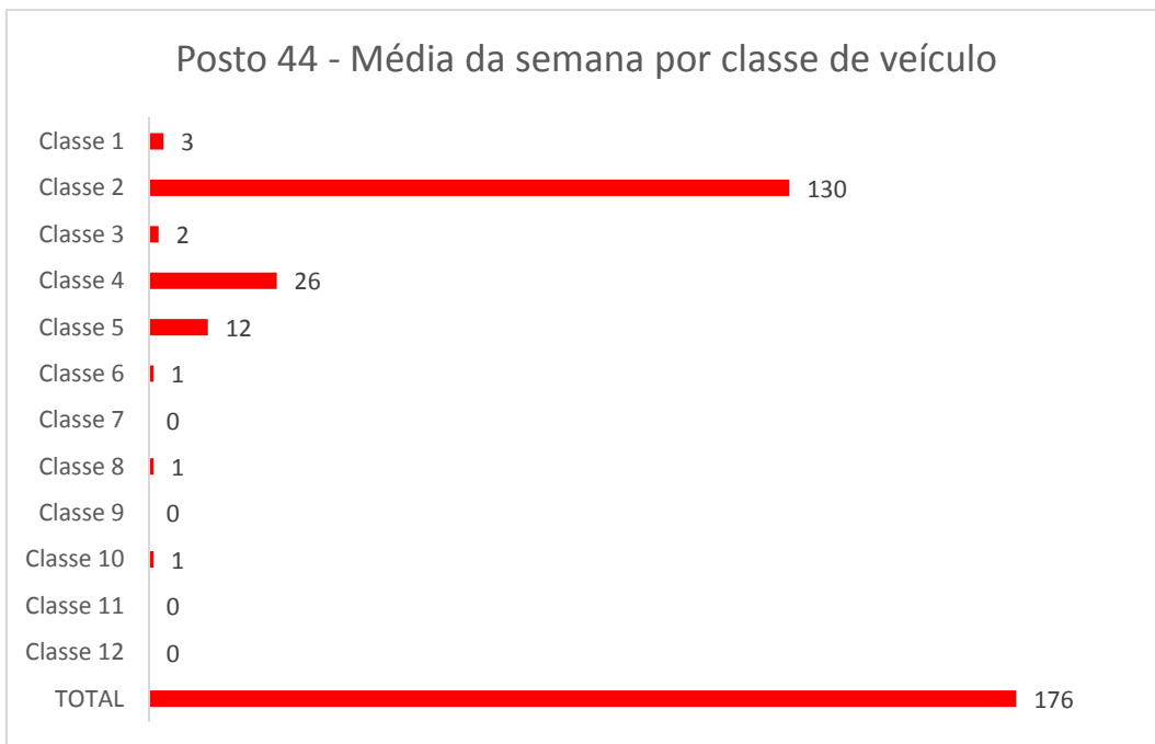
Gráfico 075: Média da semana por classe de veículo no Posto 44.
