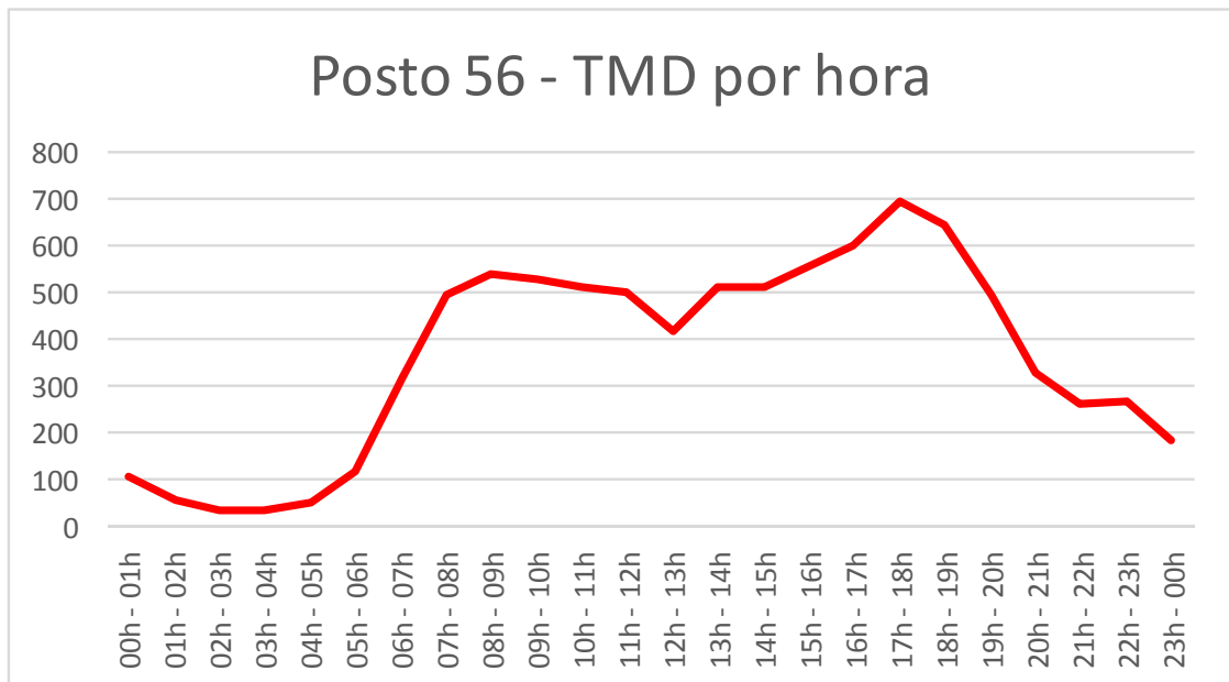
Gráfico 420: Tráfego médio diário (TMD) por hora no Posto 56.
