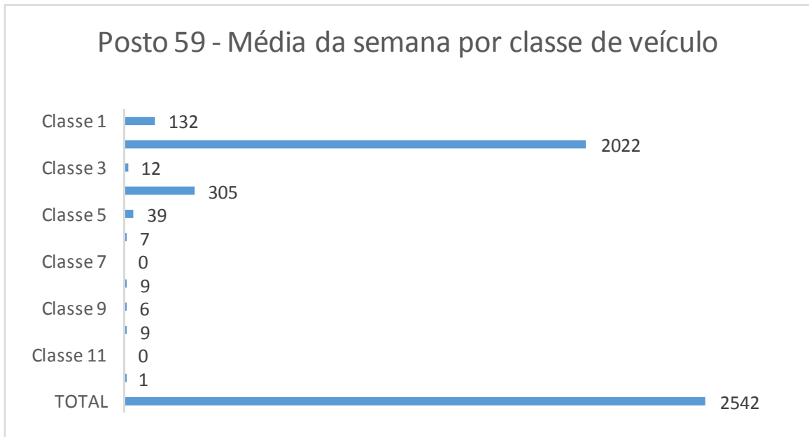
Gráfico 603: Média da semana por classe de veículo no Posto 59.
