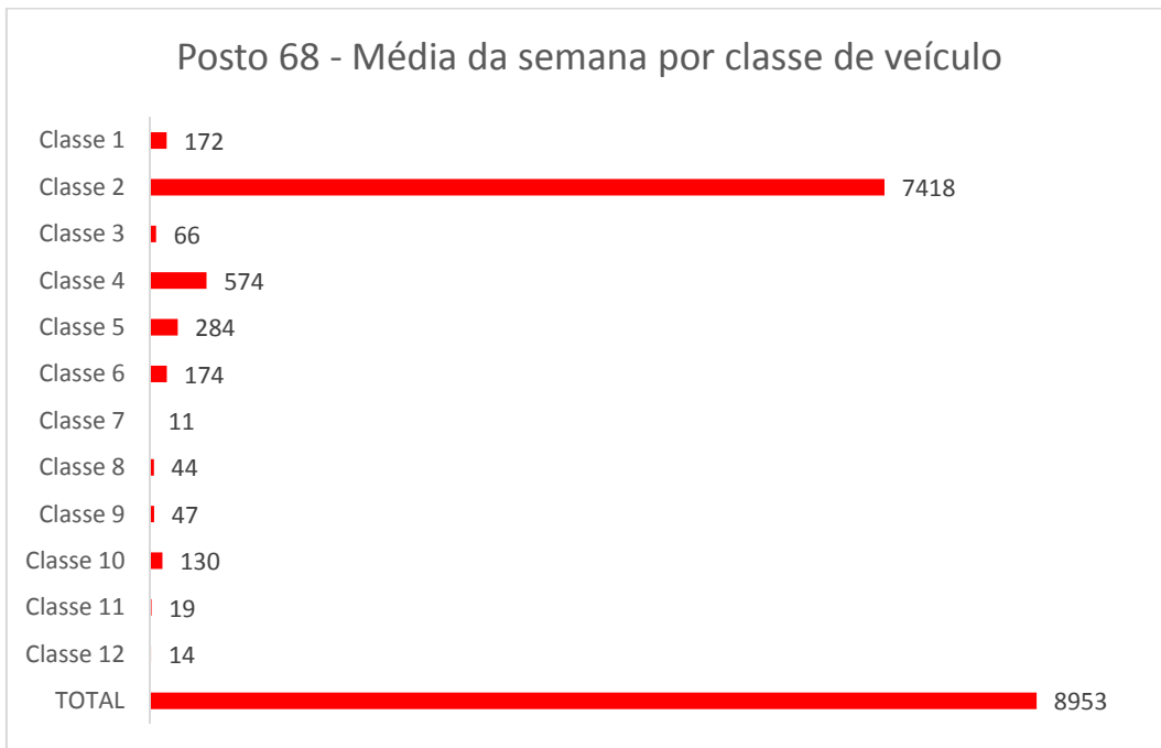
Gráfico 146: Média da semana por classe de veículo no Posto 68
