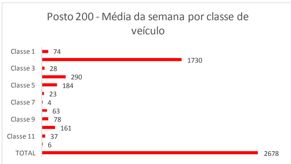
Gráfico 474: Média da semana por classe de veículo no Posto 200.
