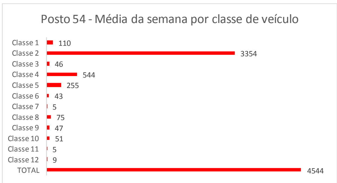
Gráfico 418: Média da semana por classe de veículo no Posto 54.
