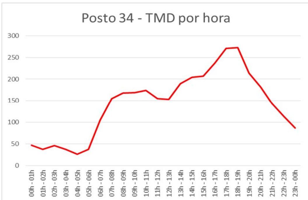
Gráfico 203: Tráfego médio diário (TMD) por hora no Posto 34.
