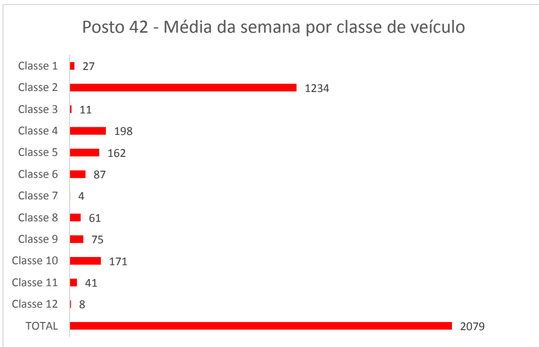
Gráfico 040: Média da semana por classe de veículo no Posto 42.
