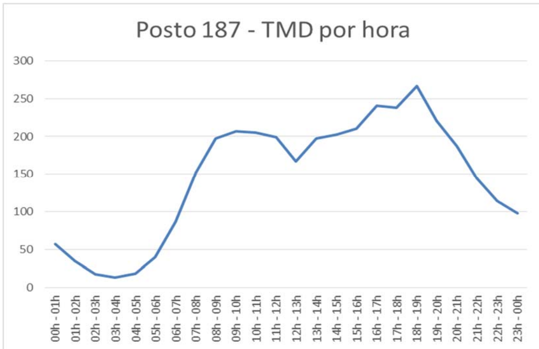
Gráfico 163: Tráfego médio diário (TMD) por hora no Posto 187
