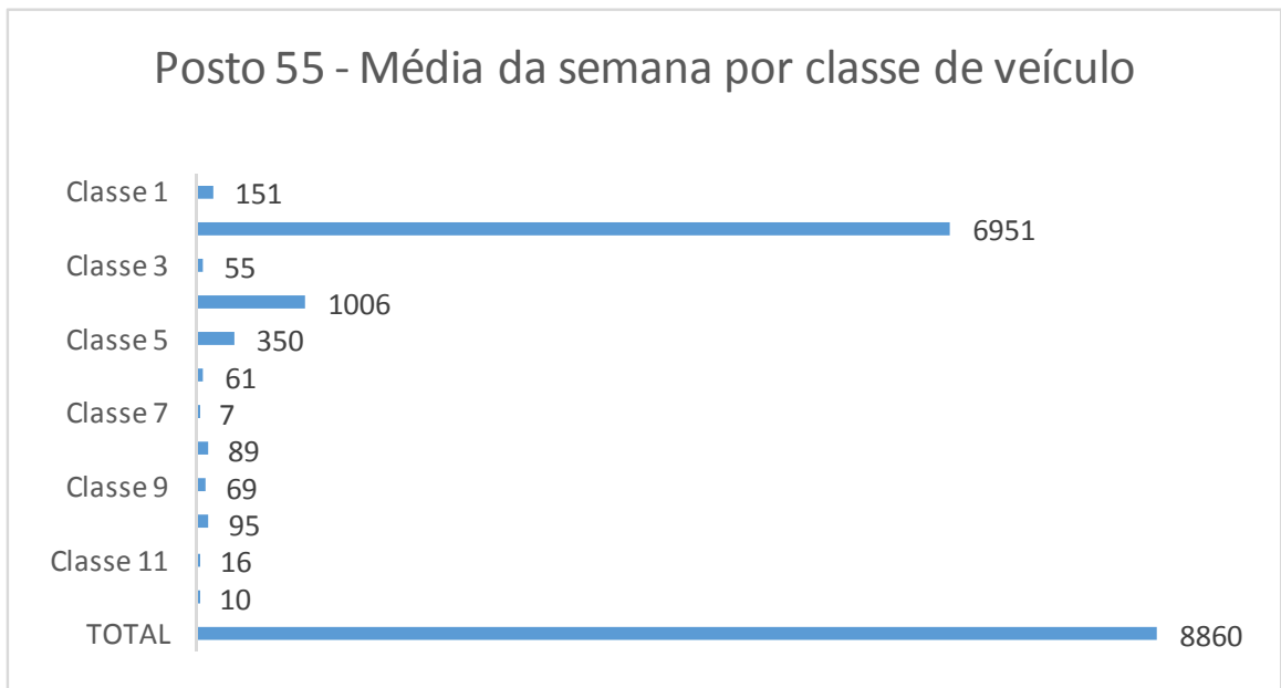
Gráfico 421: Média da semana por classe de veículo no Posto 55.
