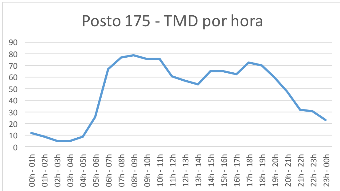
Gráfico 621: Tráfego médio diário (TMD) por hora no Posto 175.
