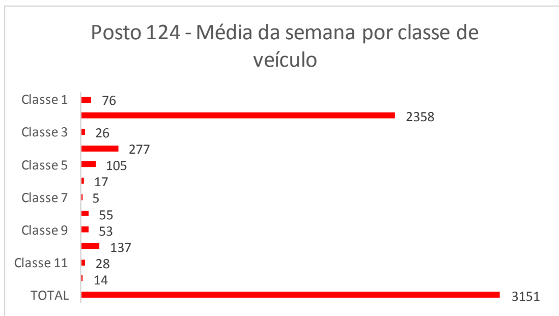
Gráfico 620: Média da semana por classe de veículo no Posto 124.
