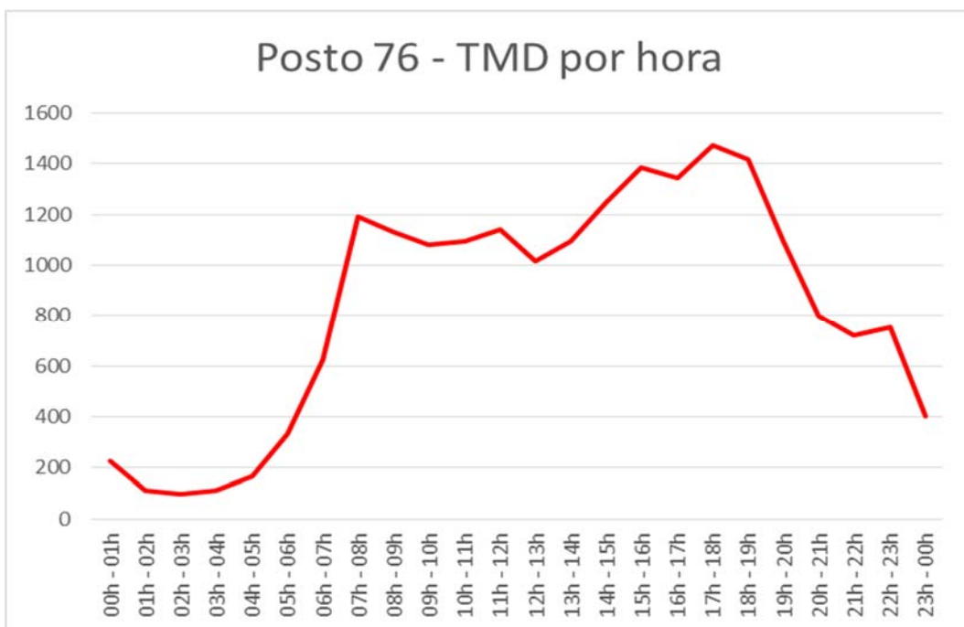
Gráfico 152: Tráfego médio diário (TMD) por hora no Posto 76
